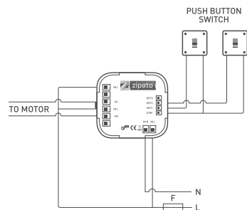
рис. 3 Соединение с двухклавишным кнопочным выключателем
