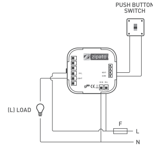
Рис. 2 Соединение с одноклавишным кнопочным выключателем
